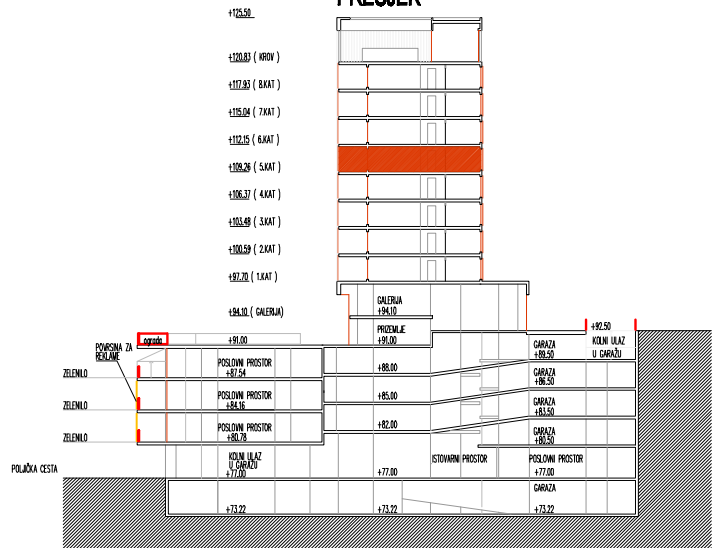
PRESJEK
