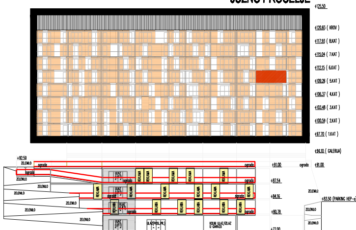
JUŽNO PROČELJE
