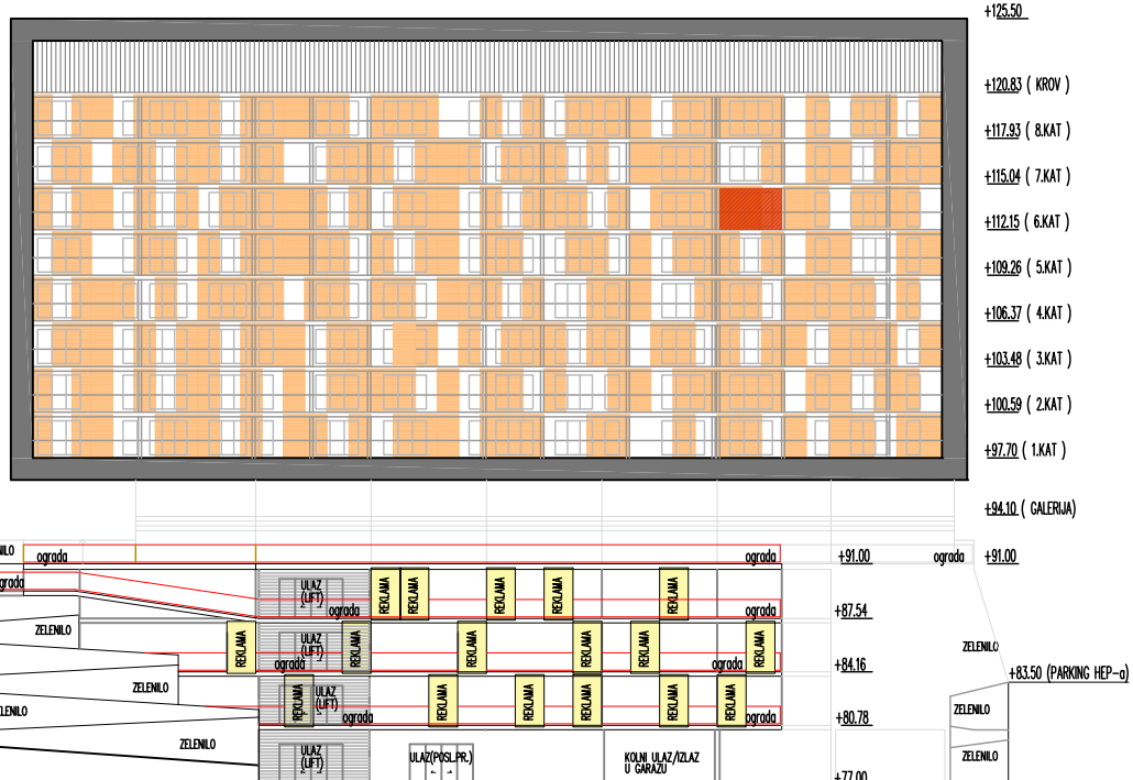
JUŽNO PROČELJE
