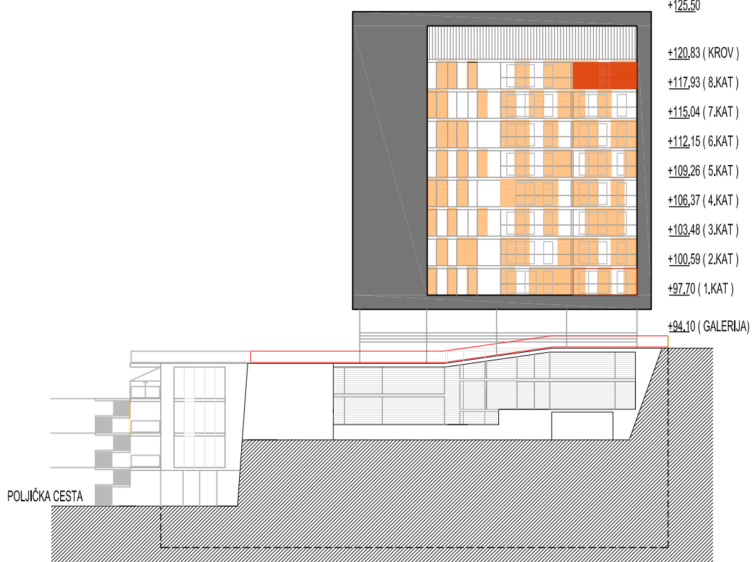
ISTOČNO PROČELJE
