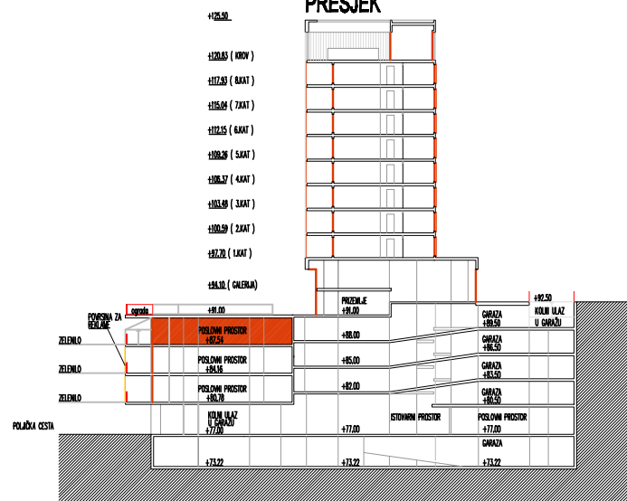
PRESJEK
