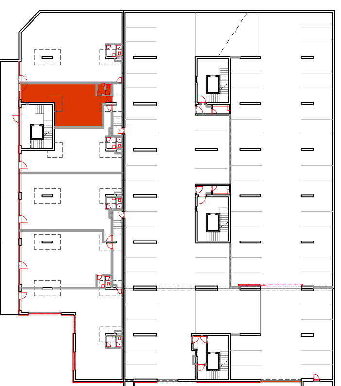
TLOCRT SUTERENA 4
