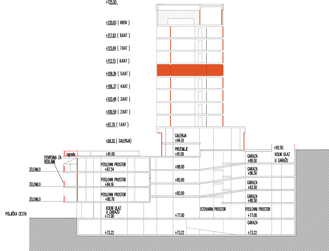
PRESJEK
