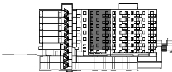
ISTOČNA FASADA
