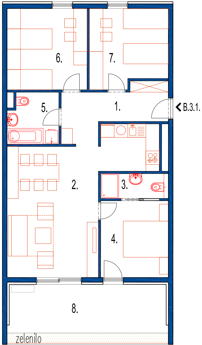
TLOCRT 3.KATA
