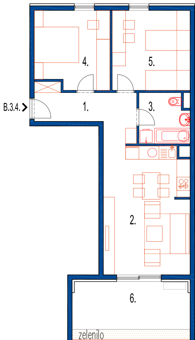
TLOCRT 3.KATA
