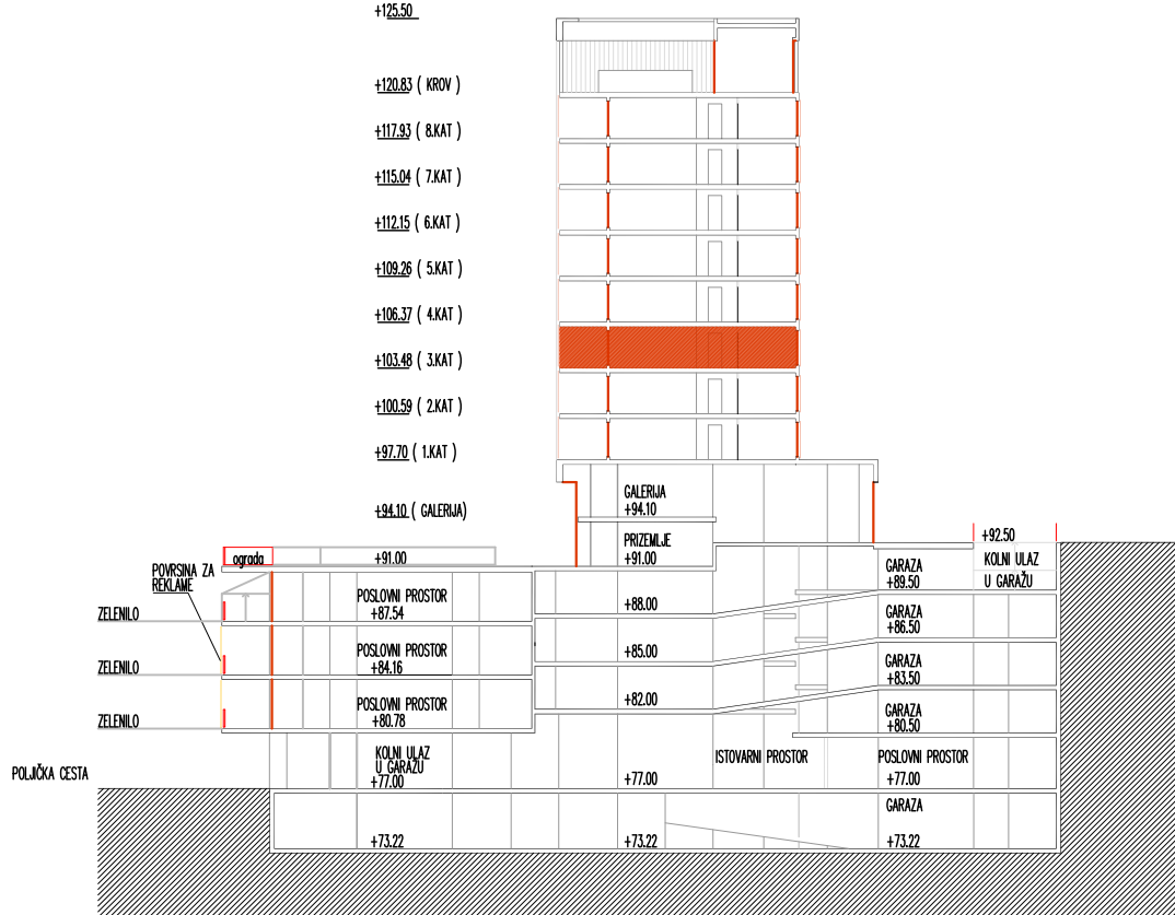
PRESJEK
