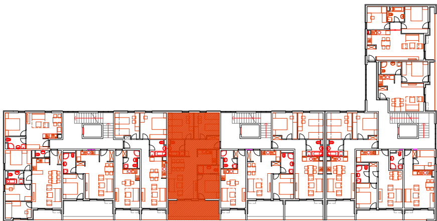
TLOCRT 6.KATA
