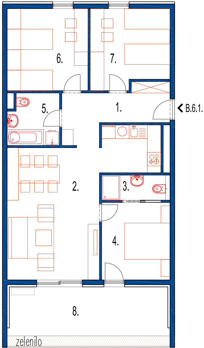
TLOCRT 6.KATA
