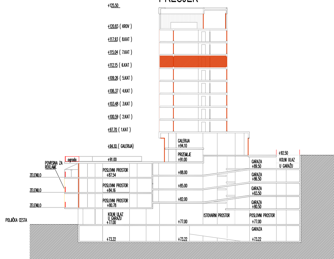
PRESJEK
