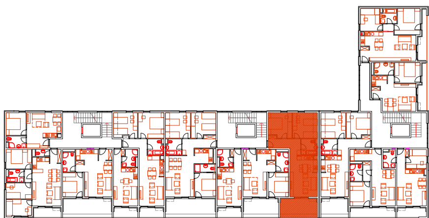
TLOCRT 7.KATA
