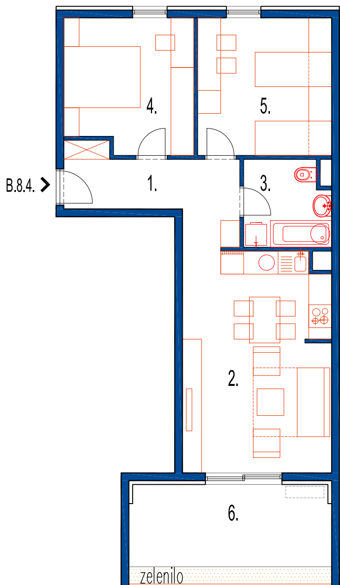
TLOCRT 8.KATA
