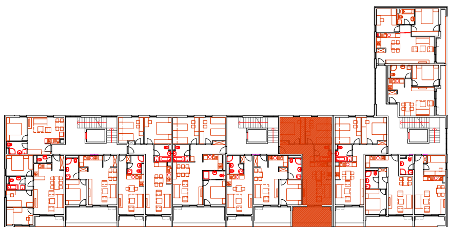
TLOCRT 8.KATA
